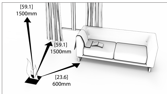
2. Dégagements Intérieur
